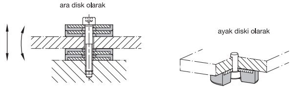
Montaj örnekleri
